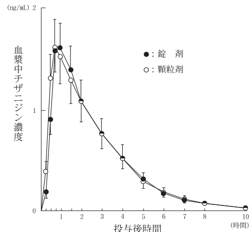
チザニジン2mg（テルネリン錠剤2錠又は顆粒剤1g）を1回投与後の血漿中濃度の推移（平均値±S.E., n=24）
