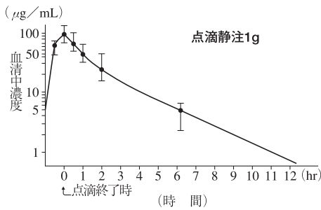
本剤1g単回点滴静注後の平均血清中濃度
